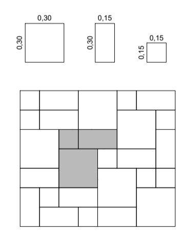
Diseño de piso 5 (DP5) Esc. 1:30
