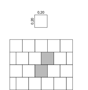
Diseño de piso 4 (DP4) Esc. 1:30
