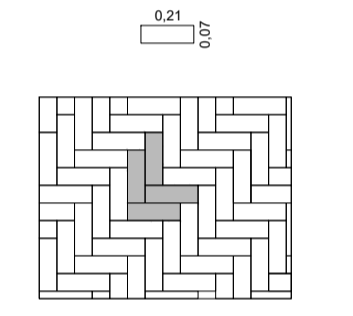
Diseño de piso 3 (DP3) Esc. 1:30
