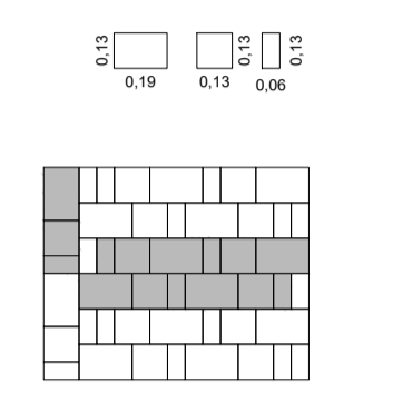
Diseño de piso 1 (DP1) Esc. 1:30
