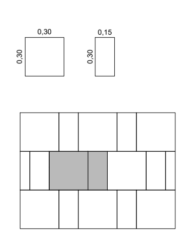
Diseño de piso 6 (DP6) Esc. 1:30
