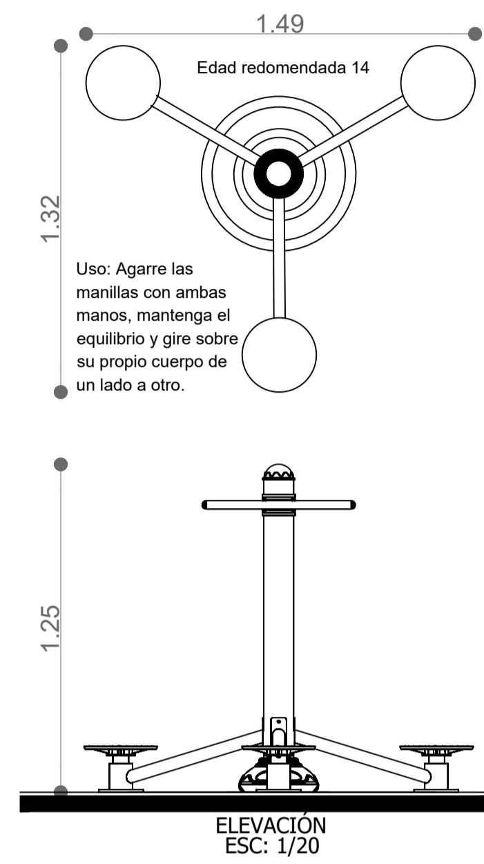
EJERCITADOR CINTURA
