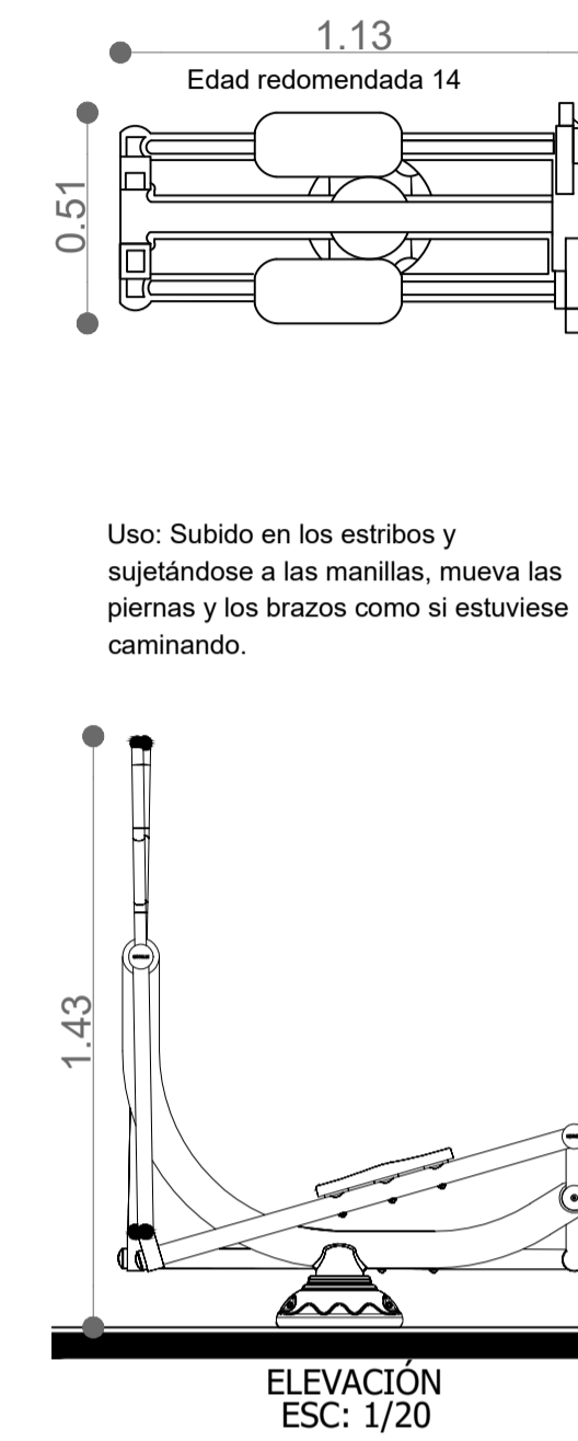
EJERCITADOR ESCALADORA
