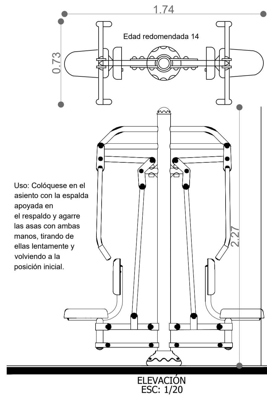
EJERCITADOR PECTORAL
