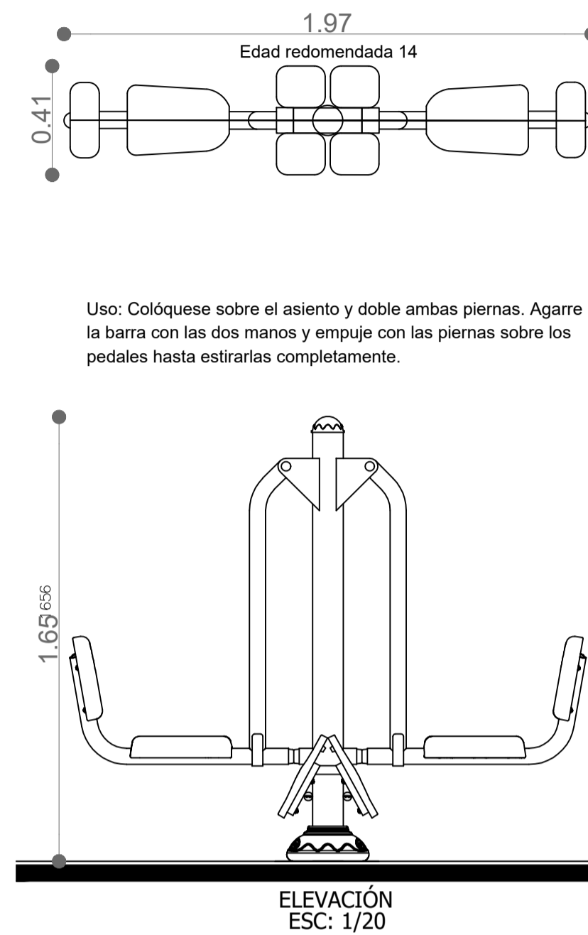
EJERCITADOR EXTENSIÓN
