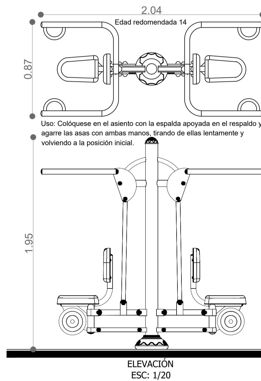
EJERCITADOR DORSALES
